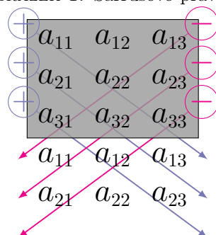
OBRÁZEK 1. Sarrusovo pravidlo
